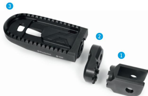
VARIO-Rastengummi »EV01«
