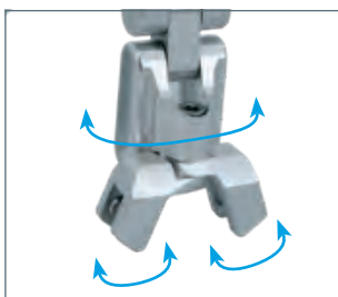
Um 180° drehbar (näher oder weiter zum Fahrer) und verstellbare Haltearme für einen spannungsfreien Sitz
